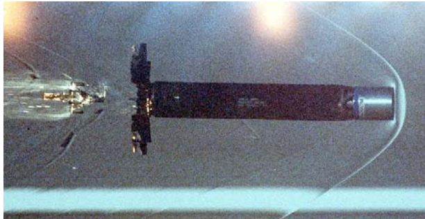
Missel com nariz achatado
